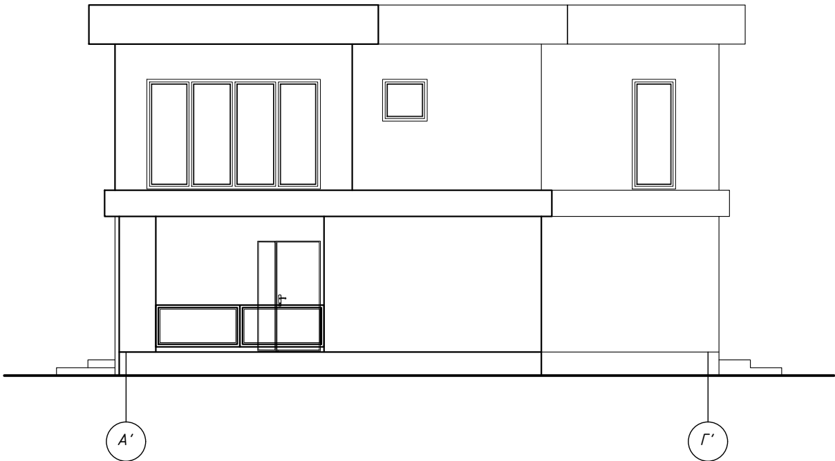
Фасад в осях А'-Г' М 1:100
